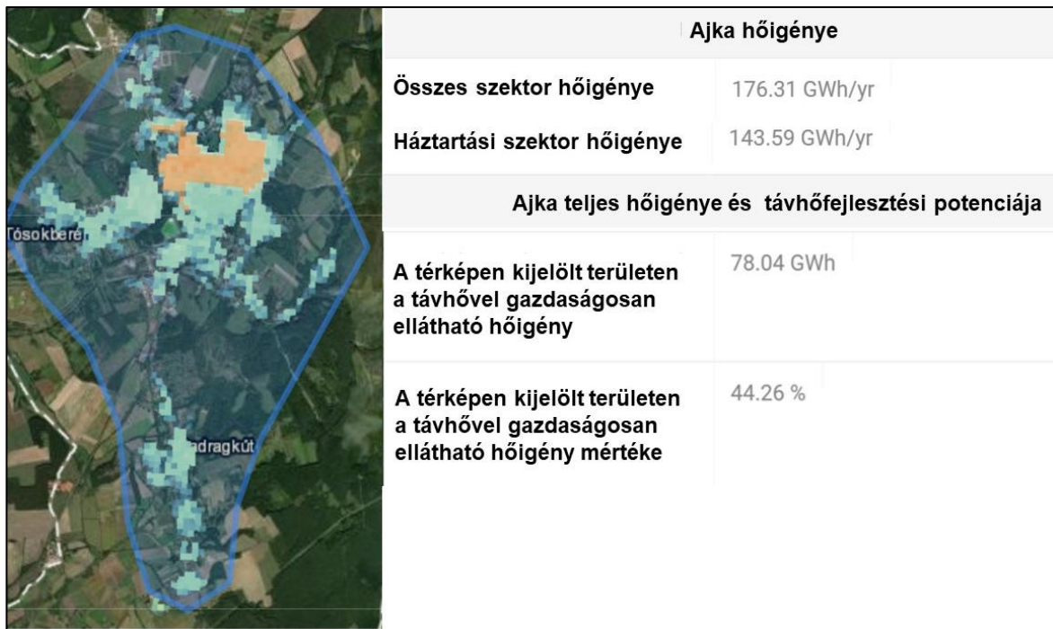
5. ábra: Ajka hőigénye, hőigénysűrűsége és prognosztizált távhő körzetei a HotMaps alapján
